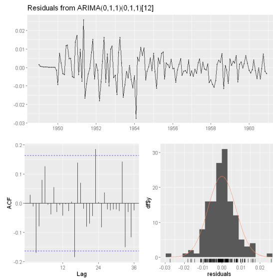
Figura 10: Gráfico de diagnóstico de resíduo
