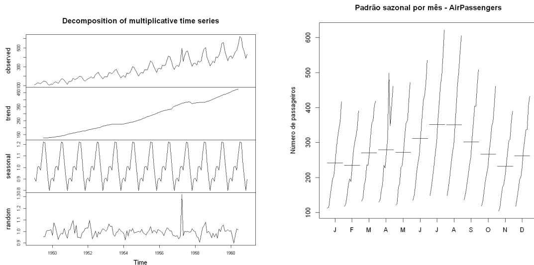
(a) Decomposição da série (b) Gráfico de sazonalidade por mês (usando monthplot)
