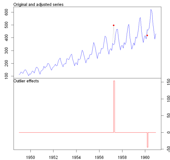
Figura 8: Série Original e a corrigida
